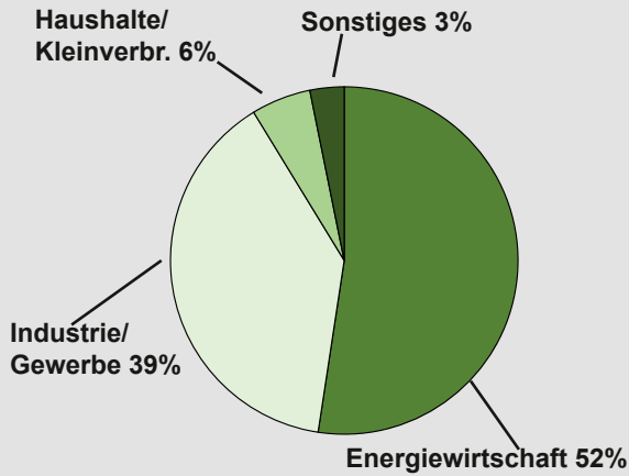
Schwefeldioxid (SO 2 )
