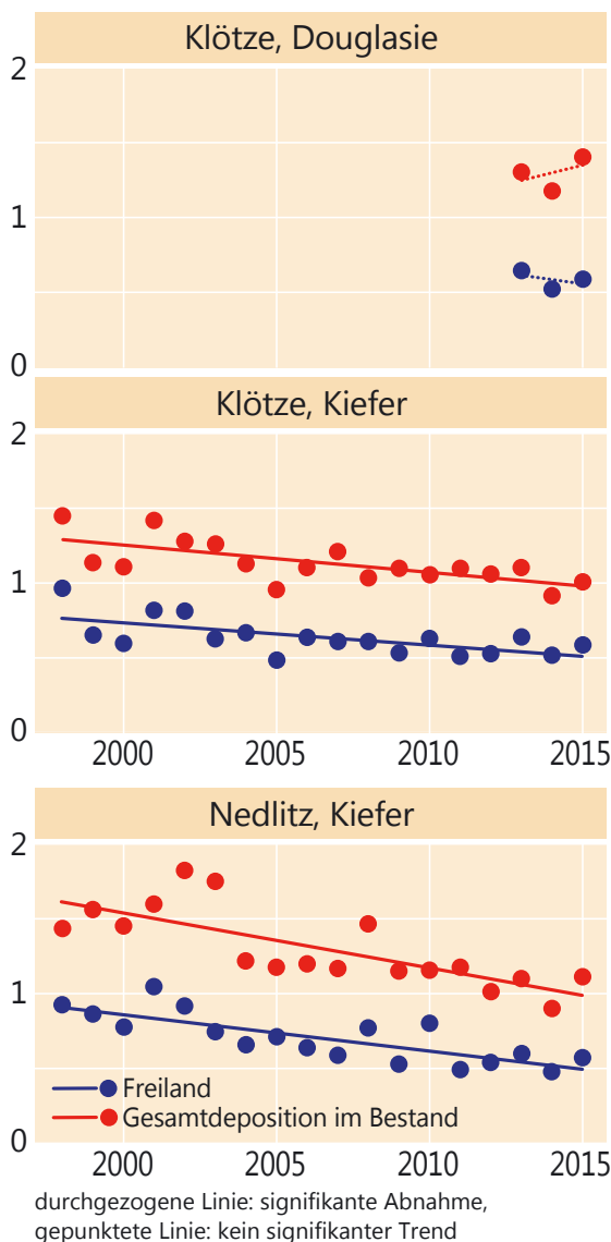
Gesamtsäure-Eintrag auf ausgewählten Flächen in kmol c je Hektar und Jahr
